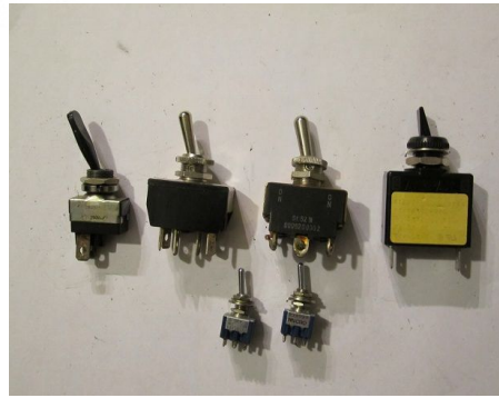
Useita virtakytkimiä
